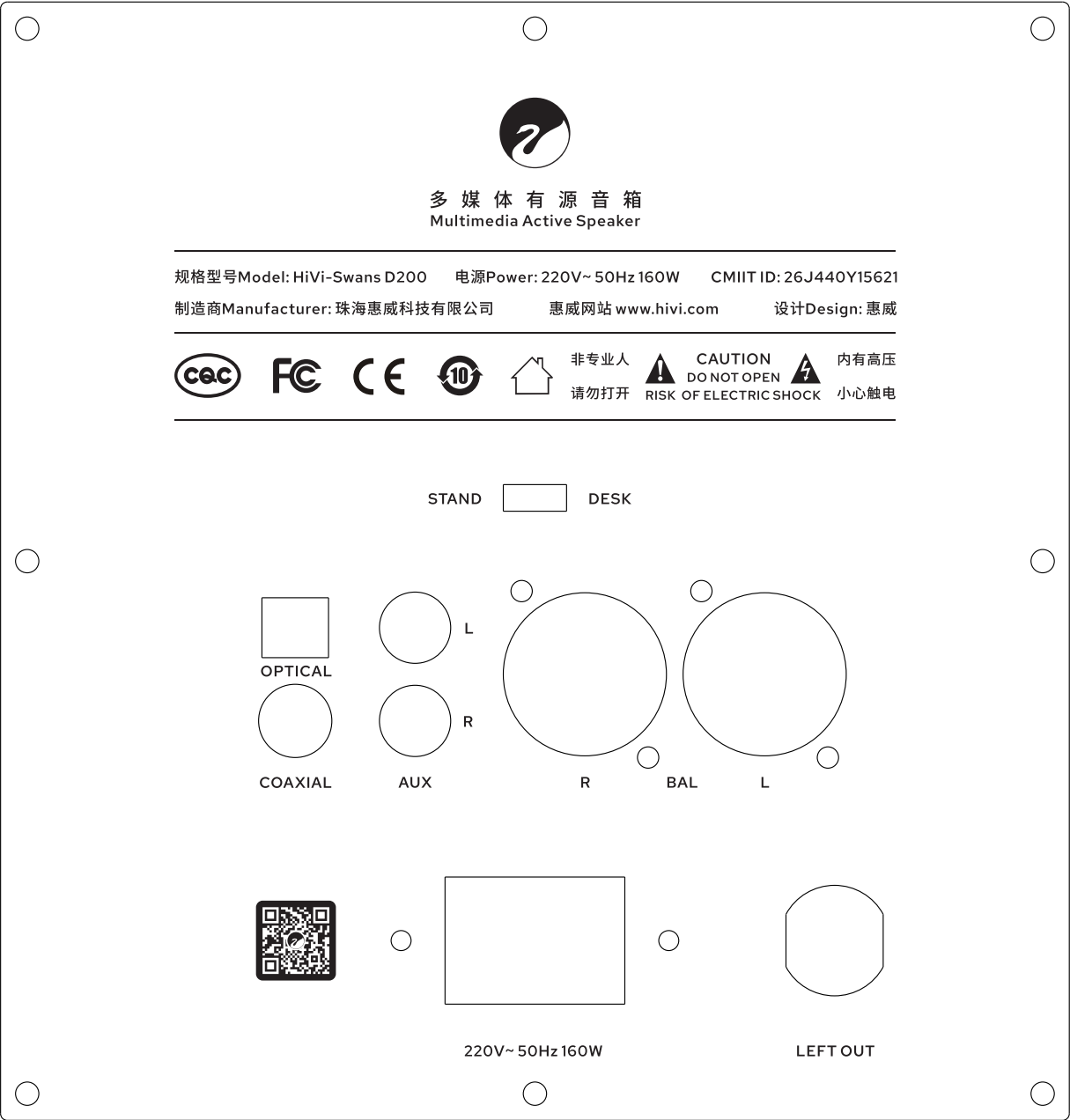
丝印位置
