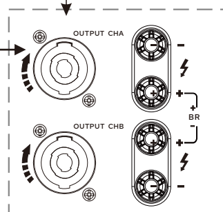
音箱螺旋插头 Speakon (NL4)
